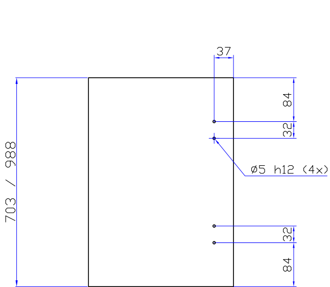
DR100D5C 703, 988 MM saranan pohjalevyn reijitys (CPK9x9, CSK-K3406X6, CSMK3406X6, L-KULMAKAAPIN ULOMMAINEN OVI ja piilonurkkakaapin peite)
