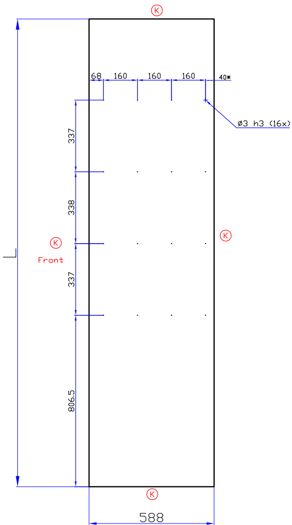
AAMIAISKAAPPI ILMAN SOKKELIA DRISAMKREV, DRISAMKREO työohjeriville merkittävä levyn koko, esim. 1920x588x16 + porauskoodi, esim. DRISAMKREV. työohjeessa ei saa olla mitään muita selityksiä tai koodeja
