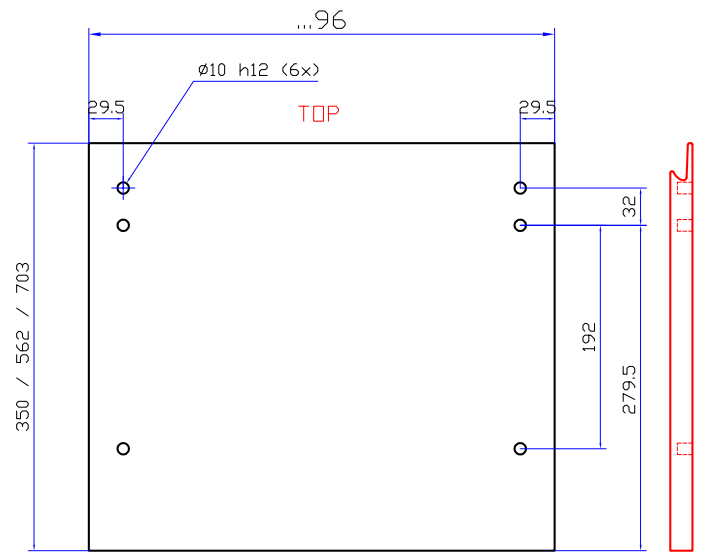
DRFBTWB 350, 562, 703 mm tandembox-jätelajittelulaatikon poraus
