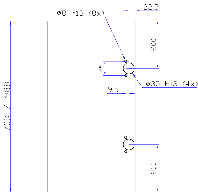
DR200D8 703, 988 mm sivusaranoidut 200 mm päästä (CSM75LT, CSM76LT, CSK95LT, CSK96LT)
