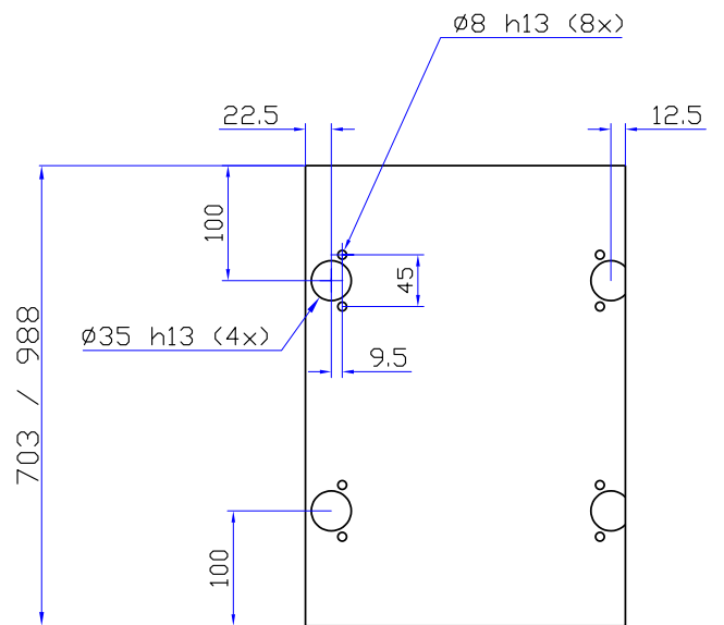
DR100D8C 703, 988 MM sivusaranoidut 100 mm päästä (CPK9x9, CSK-K3406X6, CSMK3406X6, L-KULMAKAAPIN SISIMMÄINEN OVI)
