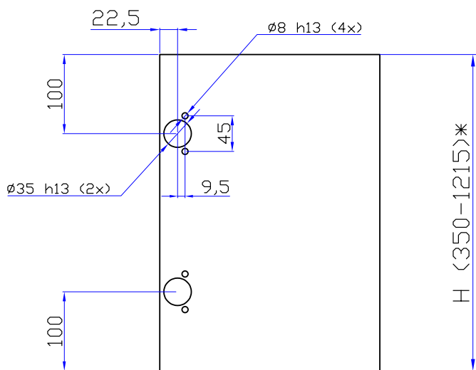
DR100D8 350-1213 MM sivusaranoidut 100 mm päästä
