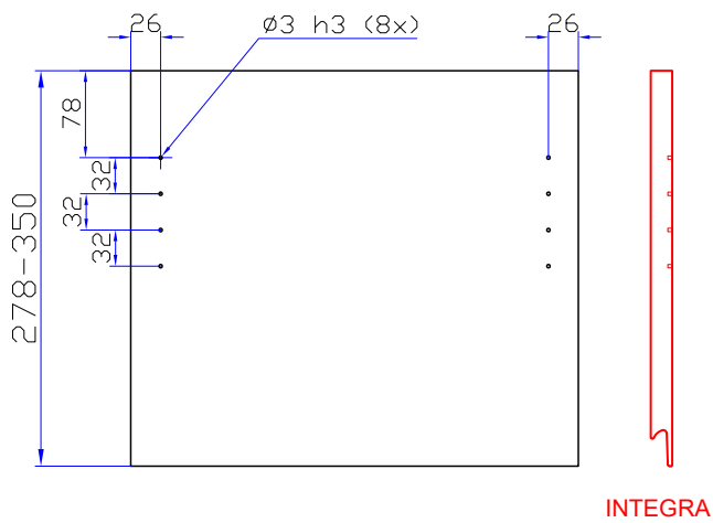
DRFBAHK 278, 350 MM kippimekanismin poraus
