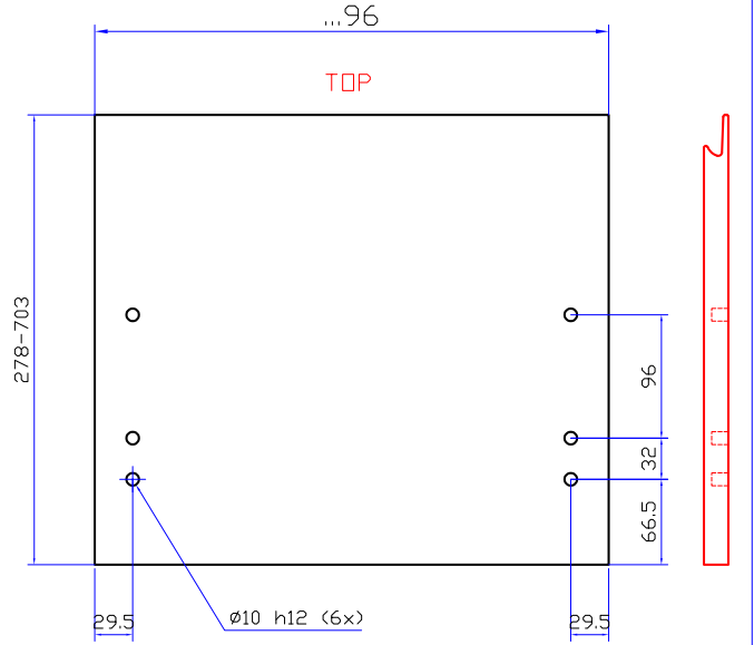
DRFBTC 278-703 MM korkean tandembox-laatikon poraus reelinkillä
