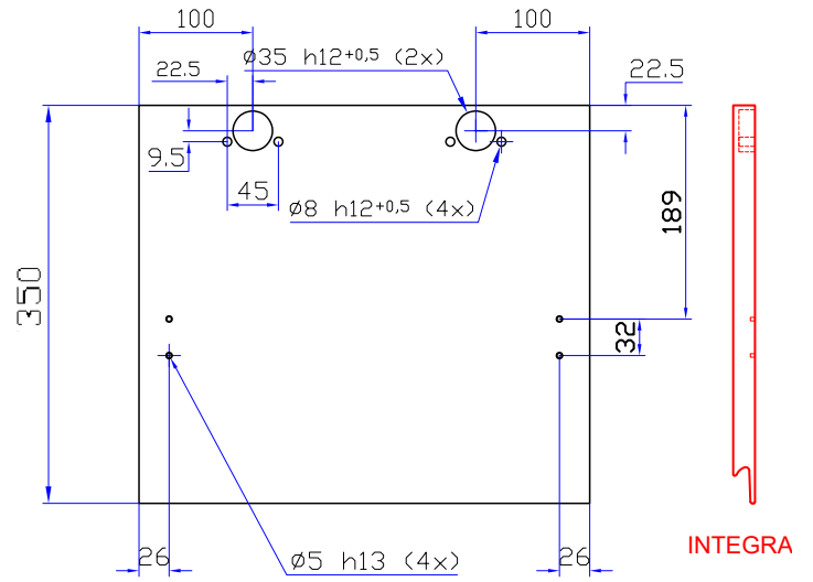
DRFBAHF2 350 MM taittomekanismin alaovi
