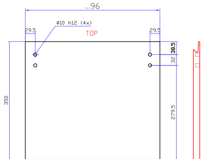
DRFBTB 350 MM tandembox-korilaatikon poraus
