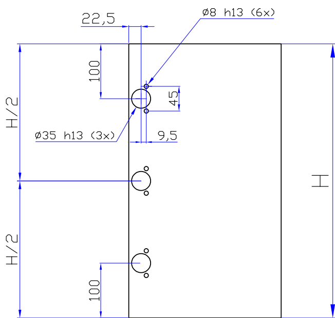
DR100D8x3 1750, 1920 mm sivusaranoidut 100 mm päästä ja yksi keskellä
