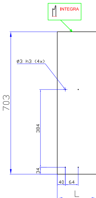
DRFPYMA 703 mm pyyhe/maustemekanismin poraus
