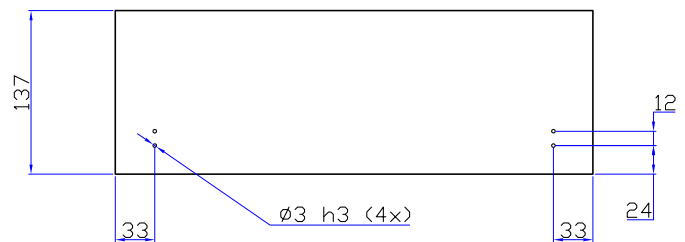
DRFLL 137 MM leikkuulaudan poraus
