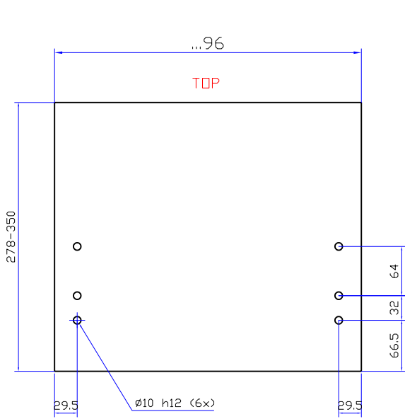
DRFBTS 278-350 MM u-tandembox-laatikon poraus reelingillä
